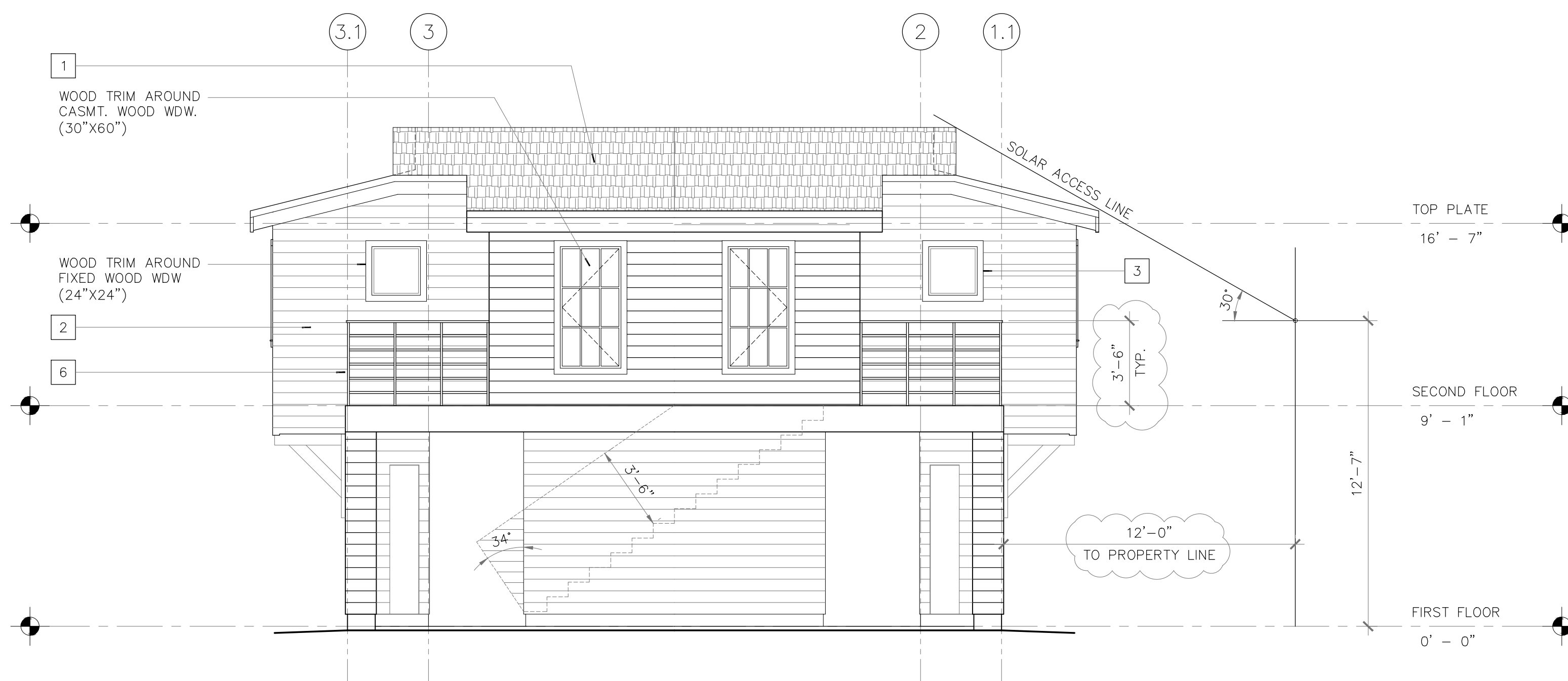
2 ELEVATION Scale: 1/4" = 1'-0"
